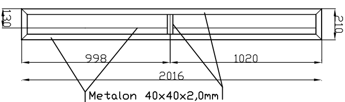
PEÇA 02 VISTA LATERAL
