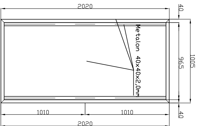
PEÇA 02 VISTA FRONTAL
