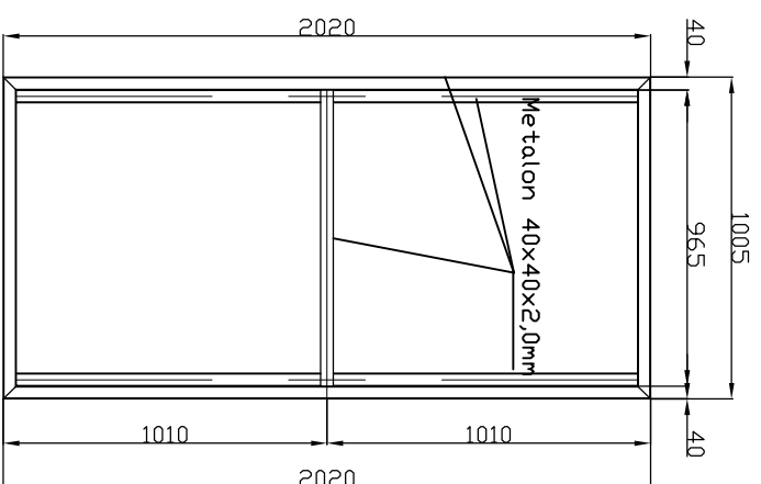
PEÇA 02 VISTA DO FUNDO
