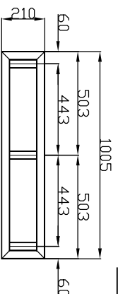
PEÇA 02 VISTA SUPERIOR E INFERIOR
